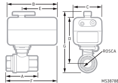
Fig. 1. Diagrama de dimensiones.
